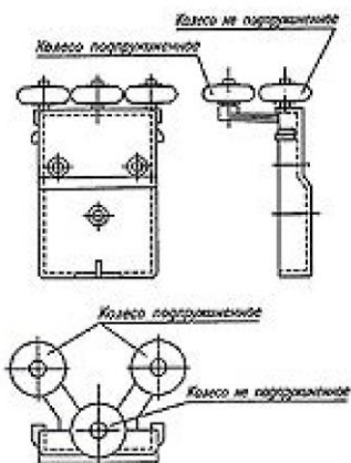
Ролик верхний
