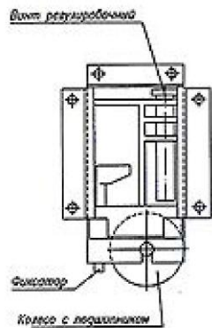
Ролик нижний
